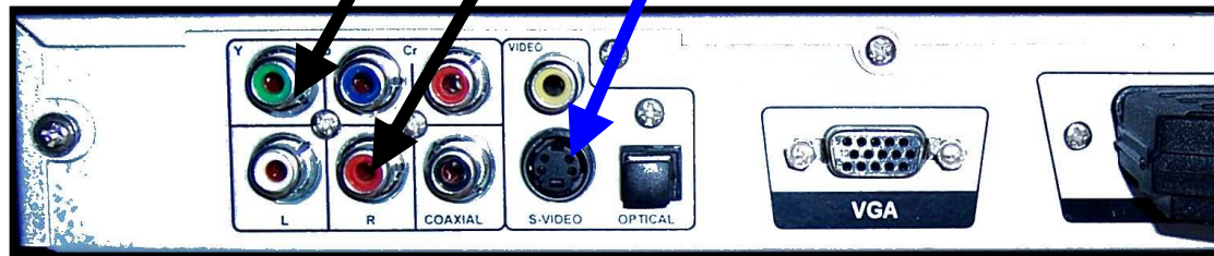
Rückseite DVD-Player Ton (L R) und Video anschließen
